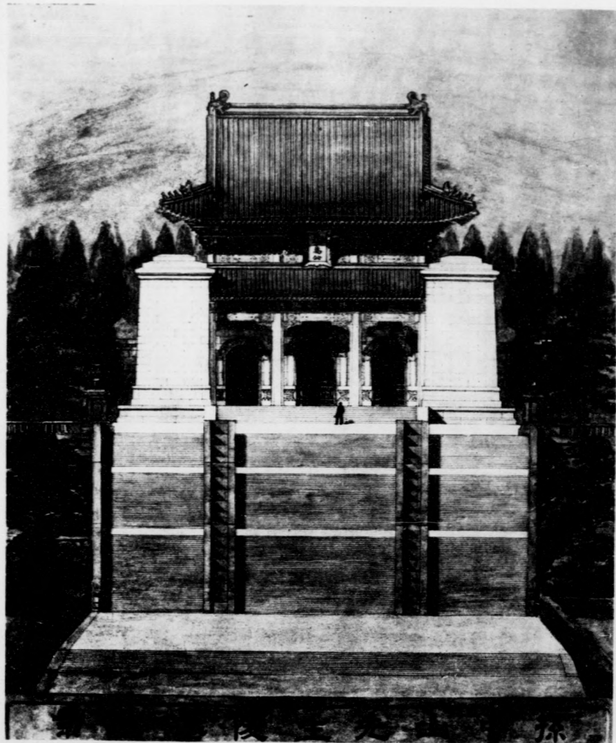
孫中山先生陵墓圖案 (二) (面正) 首獎呂彥直
